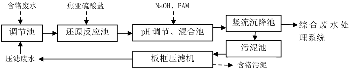
图5.2-2 含铬废水处理工艺及产污节点图
