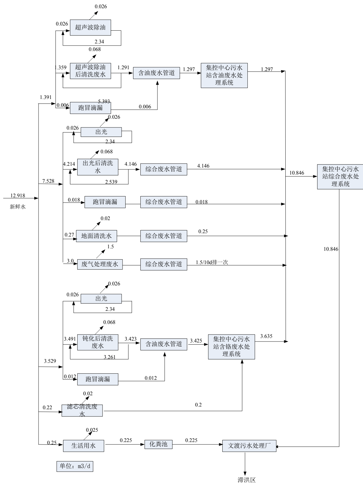
图 2.3-2 锌合金钝化日最大用水平衡图 单位: m 3 /d
