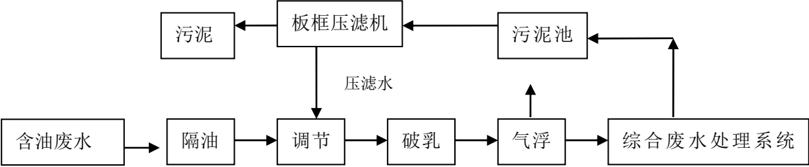
图5.2-4 含油废水处理工艺流程图
