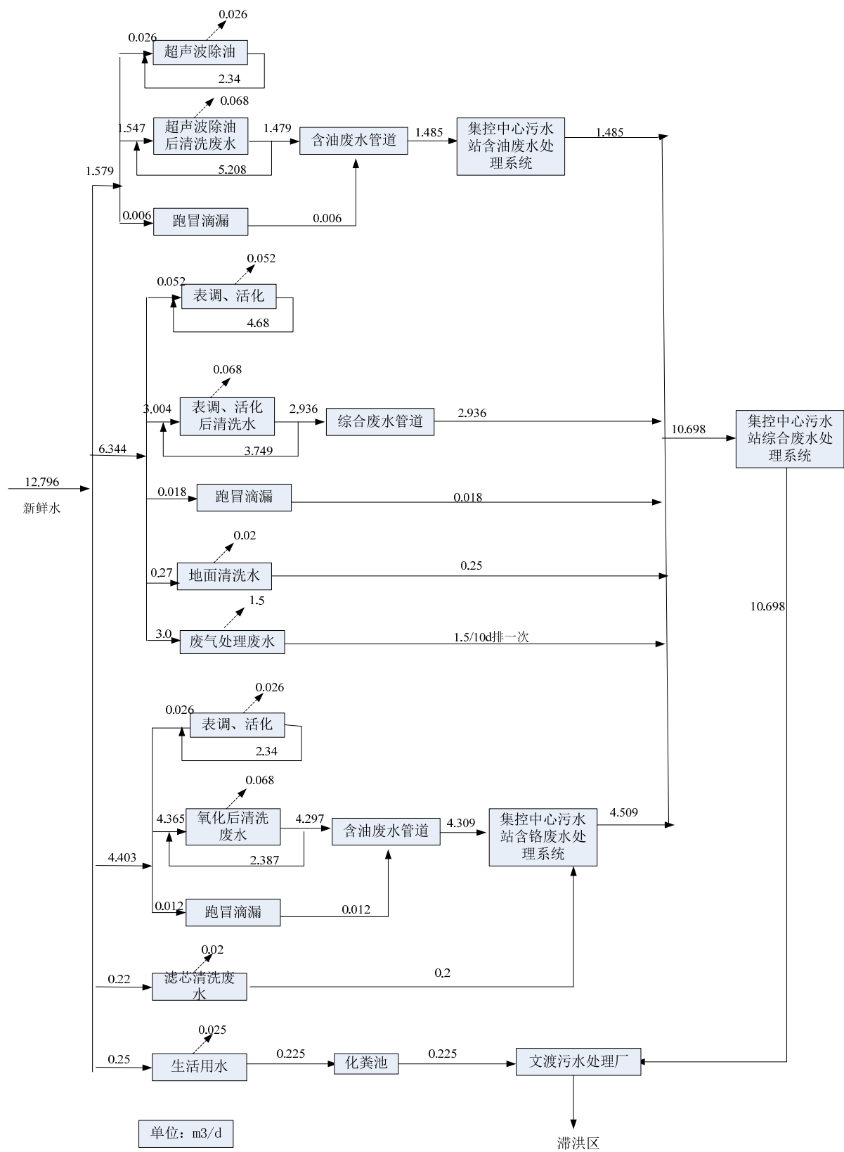
图 2.3-1 铝合金件氧化日最大用水平衡图 单位: m³/d
