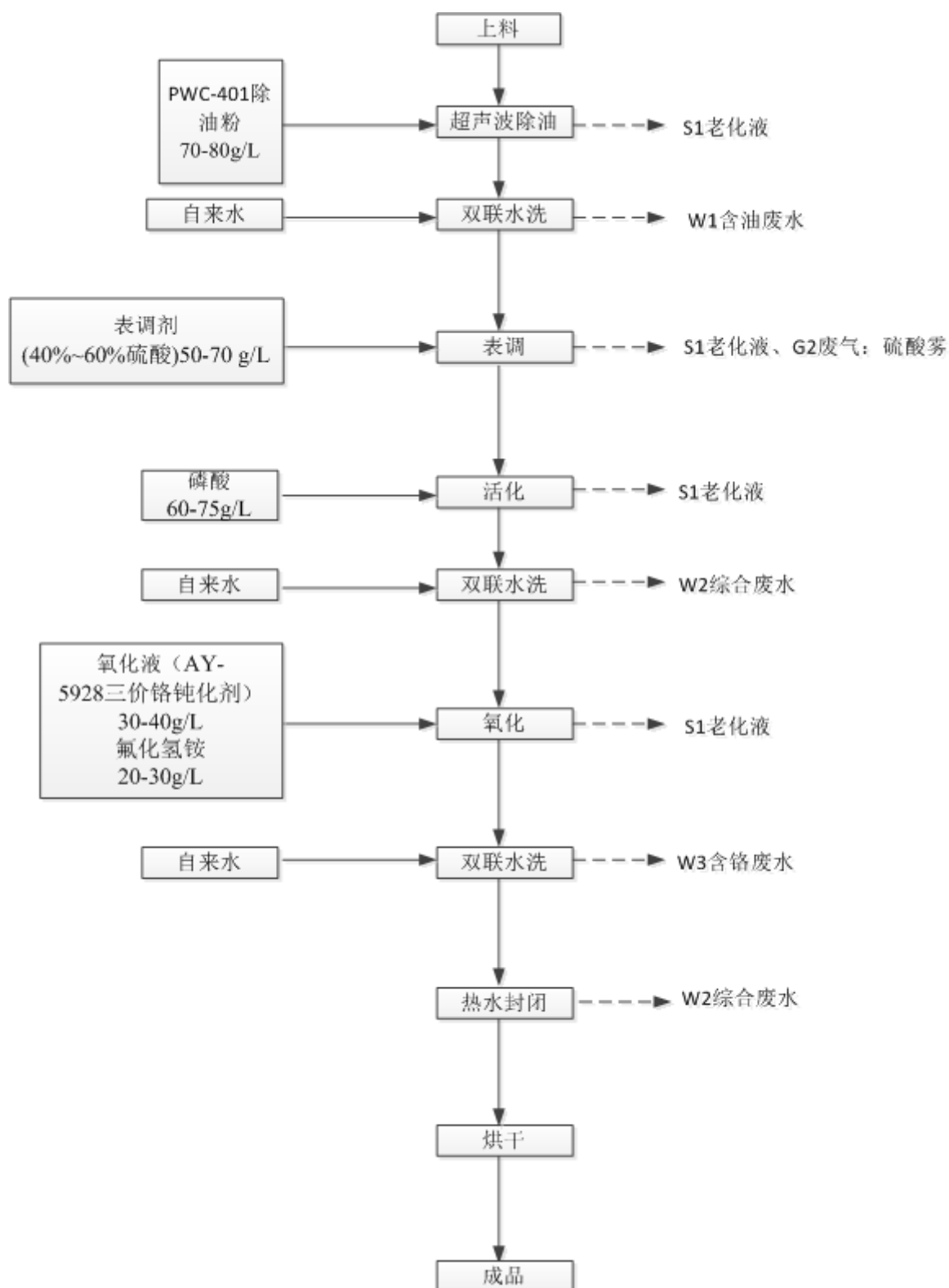
图 2.1-4 铝合金件氧化生产工艺流程及产污图
