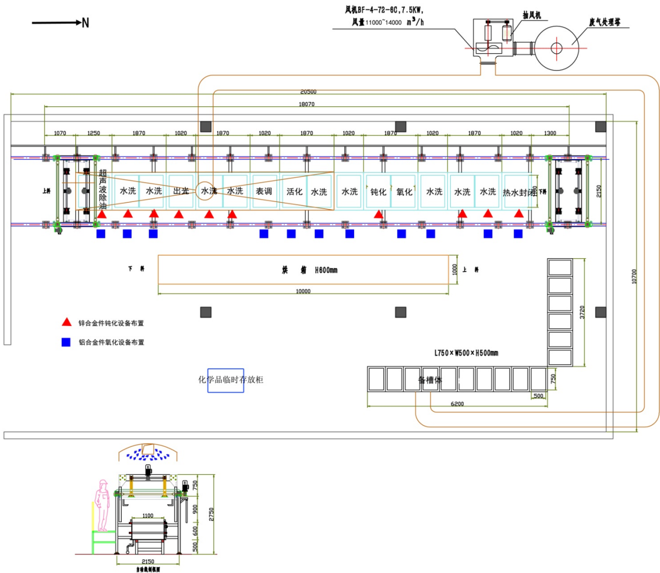
图 2.2-2 车间设备布置图
