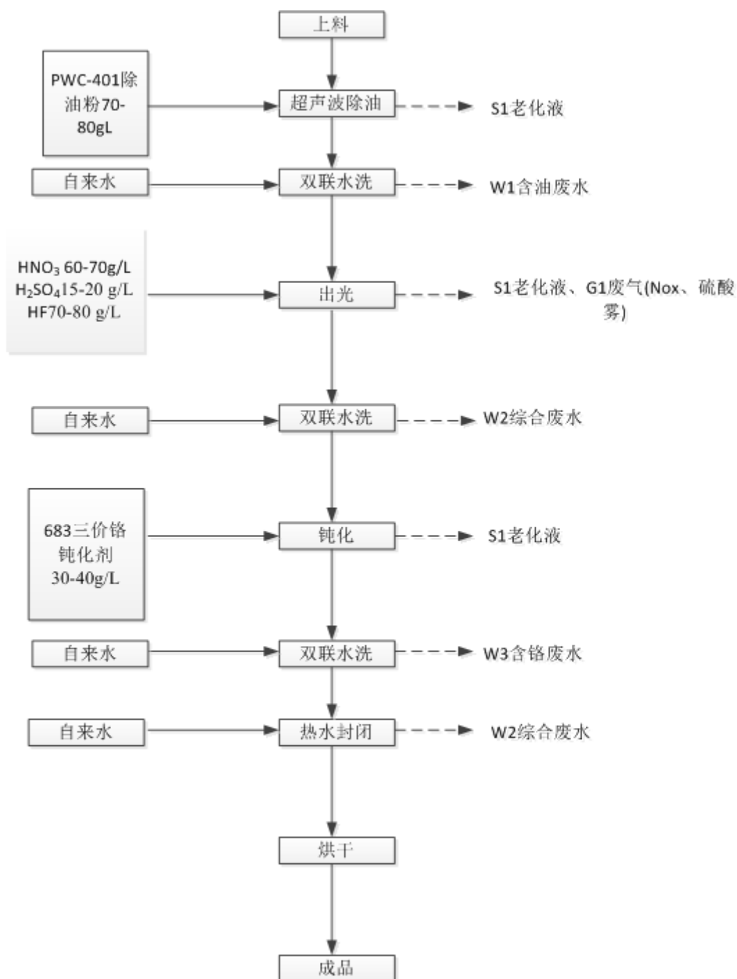
图 2.1-3 锌合金件钝化生产工艺流程及产污图
