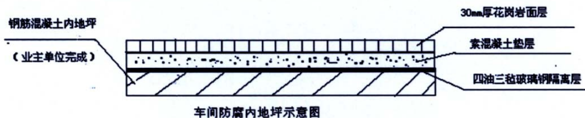
图 5.2-3 车间防渗层示意图
