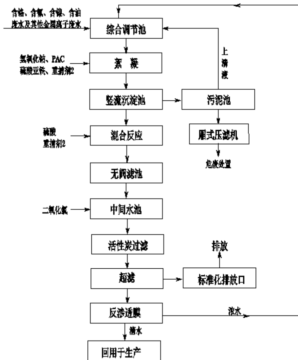
图5.2-3 含铬废水处理工艺及产污节点图
