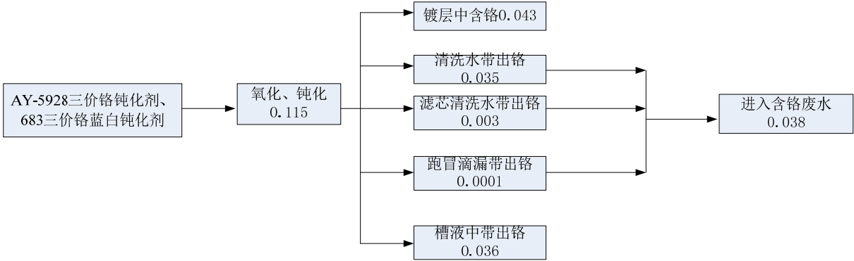
图 2.3-3 三价铬元素物料平衡图
