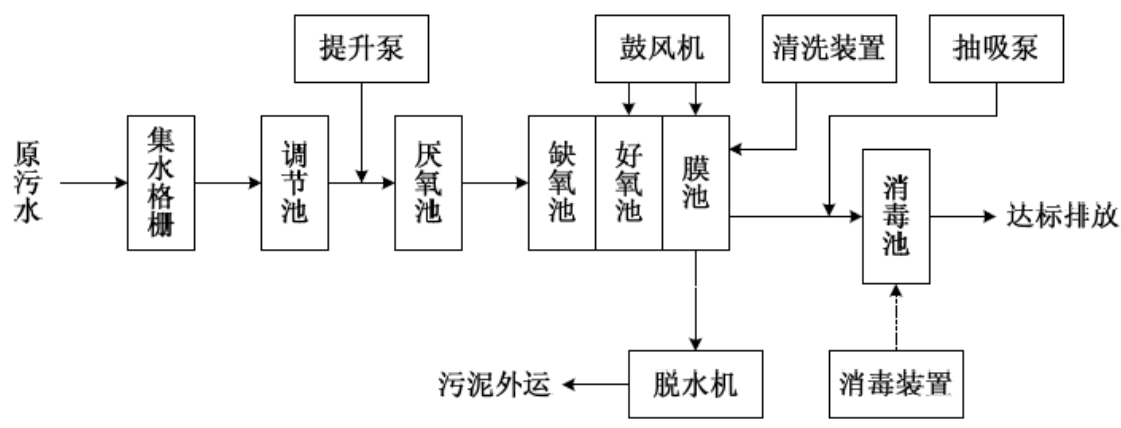
图 4.2-1 污水厂处理工艺流程图
