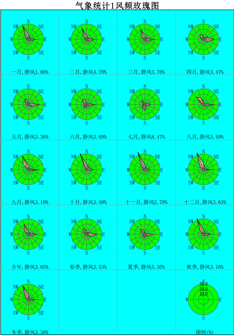
图 4.3-3 平均风速月变化图
