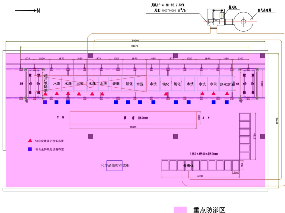
图 5.2-4 车间防渗图
